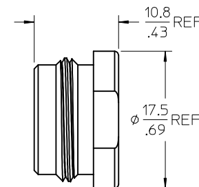
CLAMP NUT
