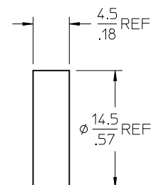
GASKET
