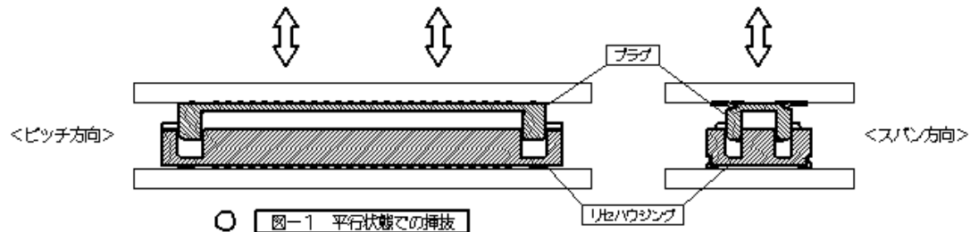
○ 図-1 平行状態での挿抜 Fig.1
