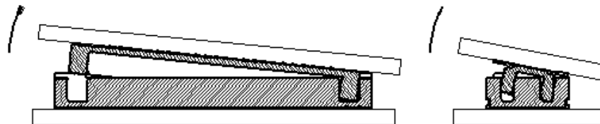
× 図-5 こじり抜去 Fig.5
