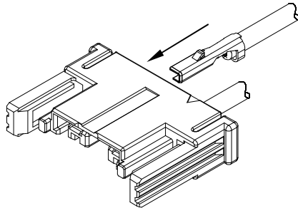
<図1 端子挿入方向>
