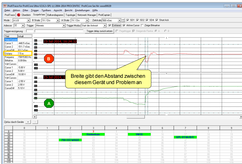
Abb. 13 - Kurzschluss (B-Schild) A&B
