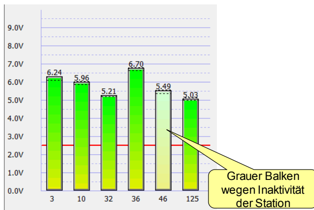
Abb. 5 - Inaktive Station im Balkendiagramm
