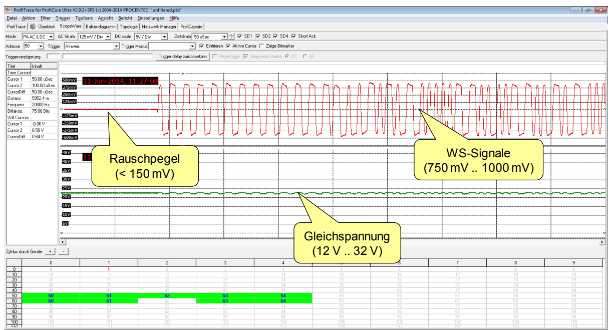
Abb. 45 - Gleichspannungs- und Wechselspannungsmessung
