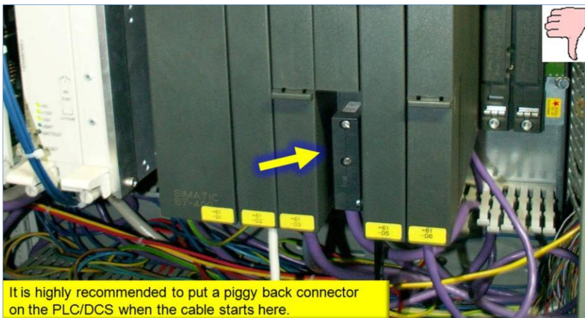
Abb. 19 - Segment ohne Huckepack-Stecker
