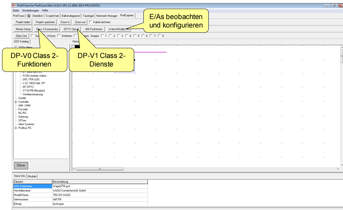
Abb. 29 - ProfiCaptain-Spezialfunktionen
