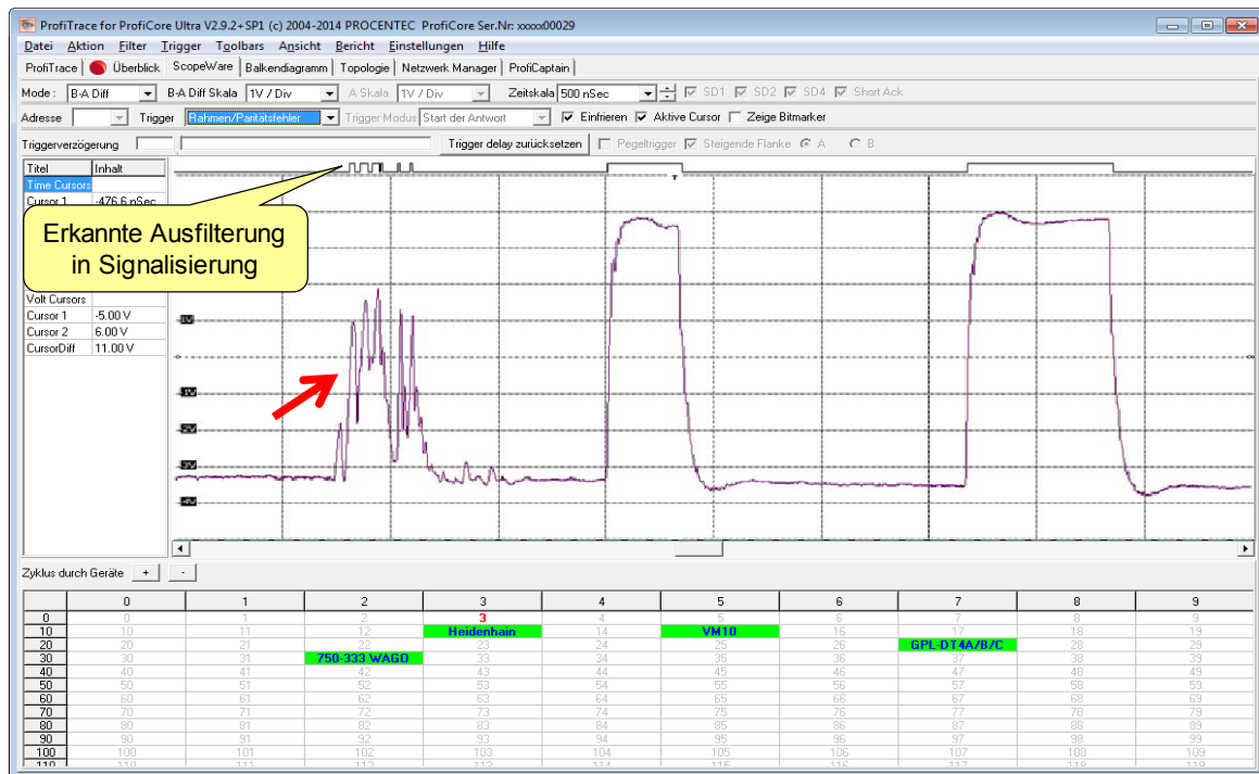
Abb. 43 - EMC/EMI-Störungen
