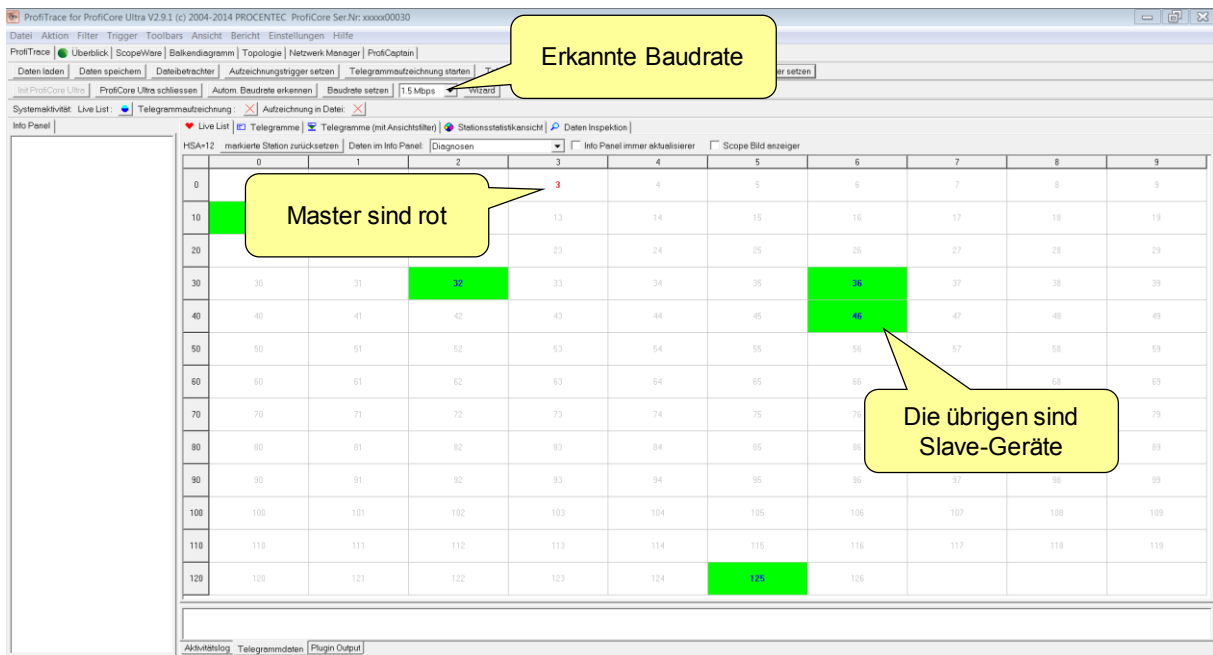
Abb. 13 - Live List nach der Initialisierung
