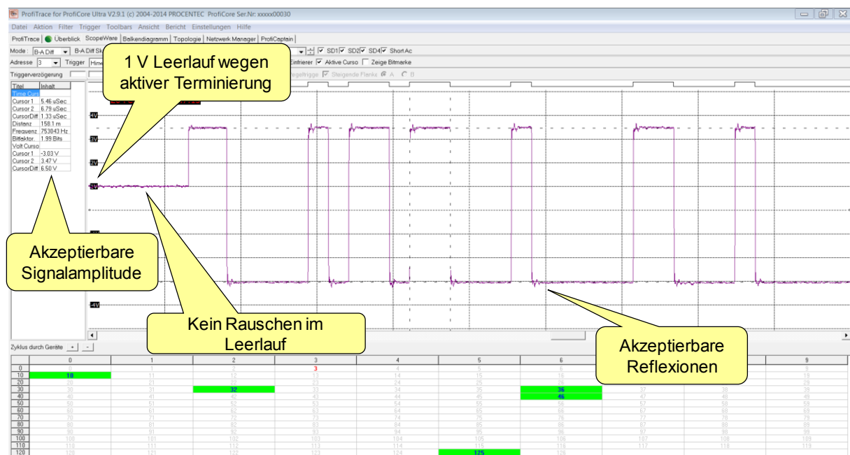
Abb. 36 - Akzeptierbare Signale bei RS 485 – DP
