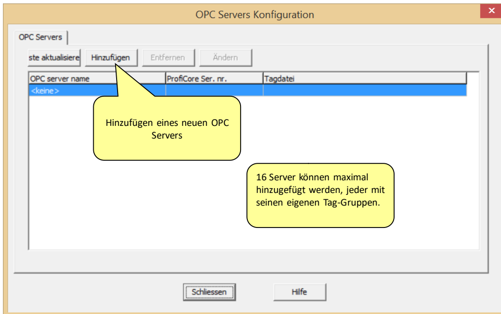
Abb. 51 - OPC-Server hinzufügen
