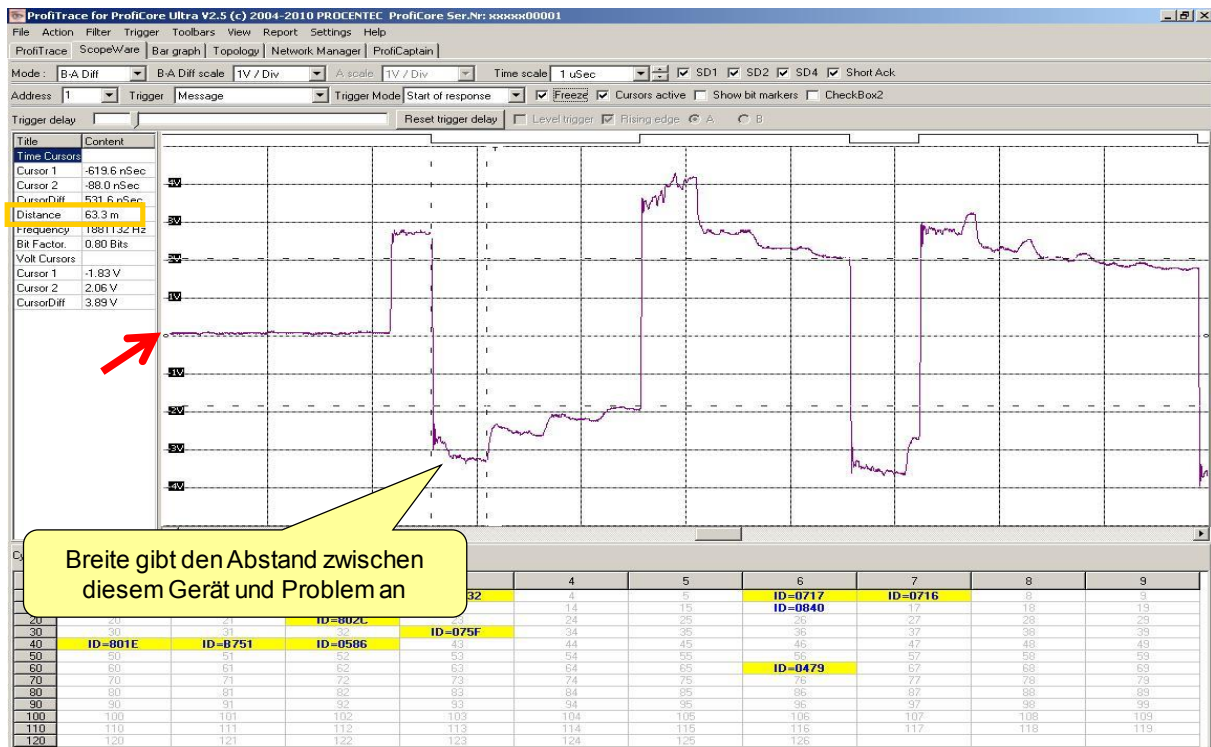
Abb. 12 - Kurzschluss zwischen A- und B-Leitung
