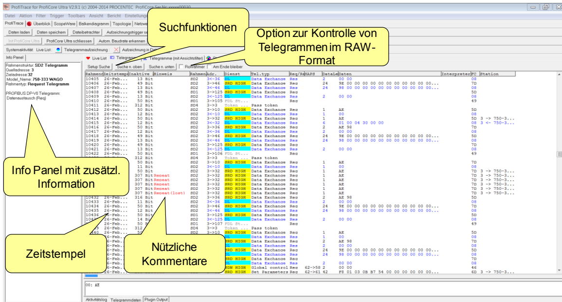
Fig. 19 - ProfiTrace Telegrammaufzeichnung
