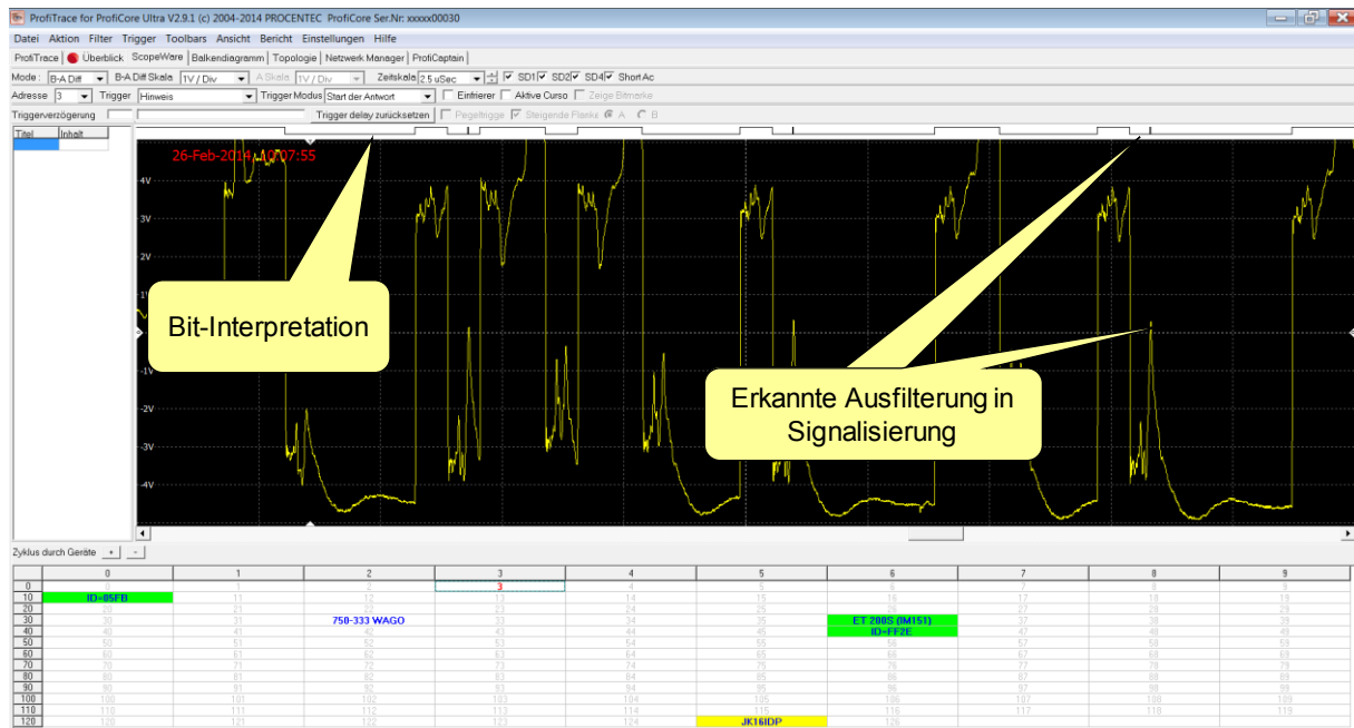
Abb. 21 - Bit-Interpretation
