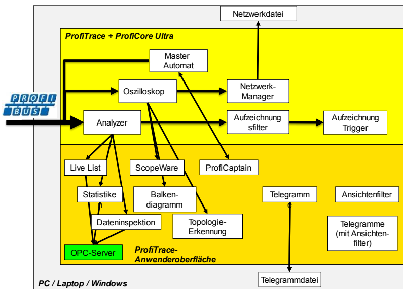
Abb. 1 - ProfiTrace-Prozesse
