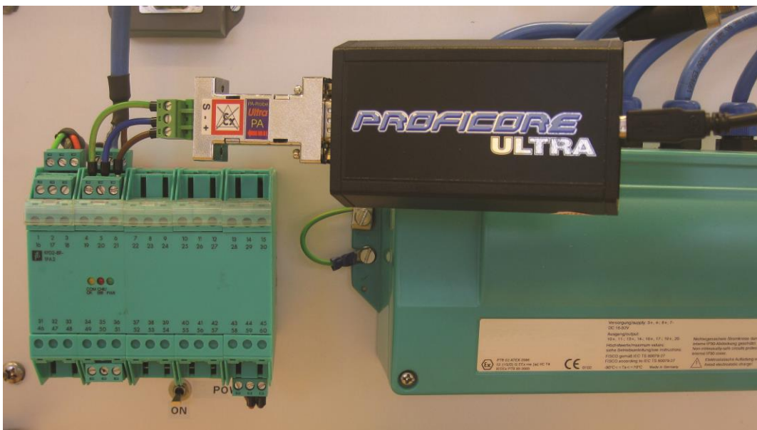
Abb. 11 - PA Probe an die Installation anschließen
