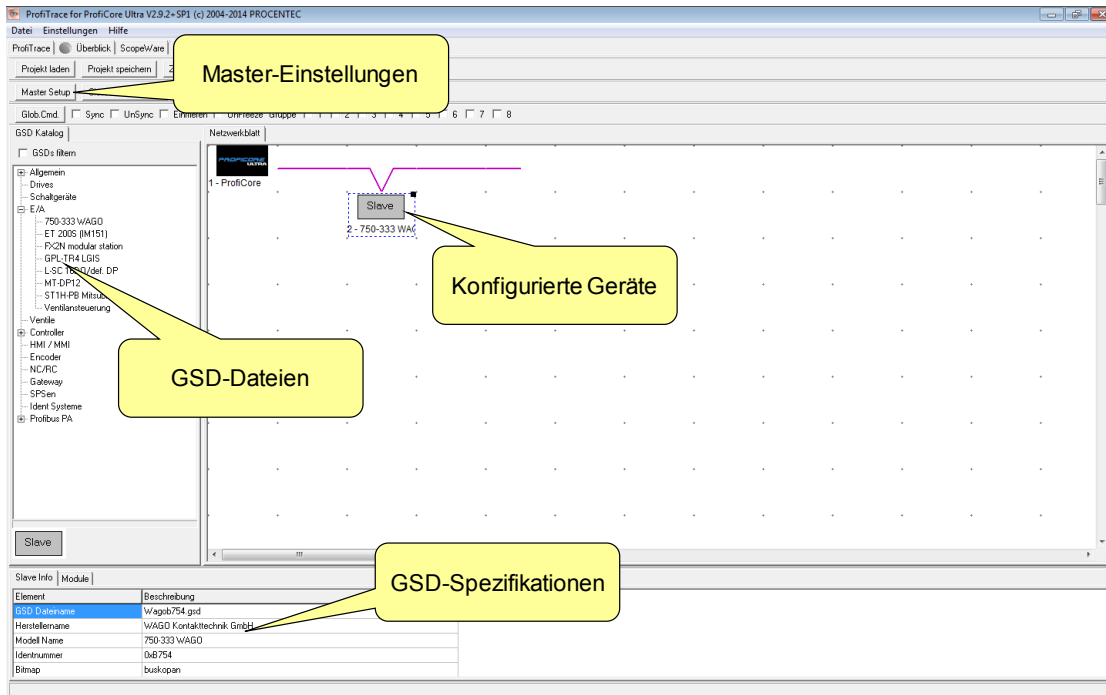
Abb. 28 – ProfiCaptain-Spezialfunktionen
