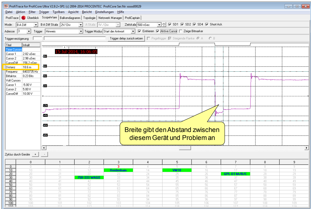
Abb. 41 - Zu viel Terminierung
