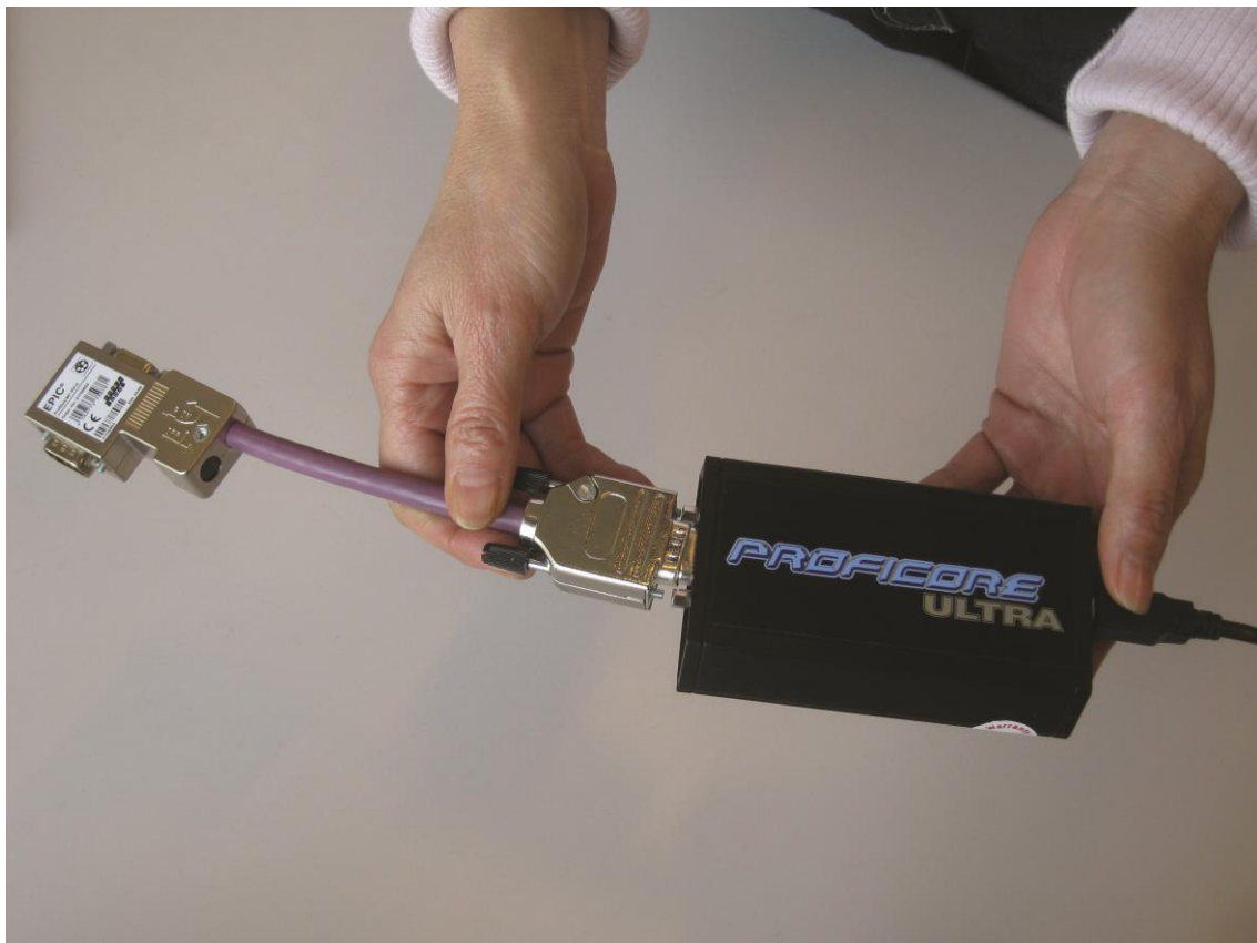
Abb. 8 - Tap Connector an den ProfiCore anschließen
