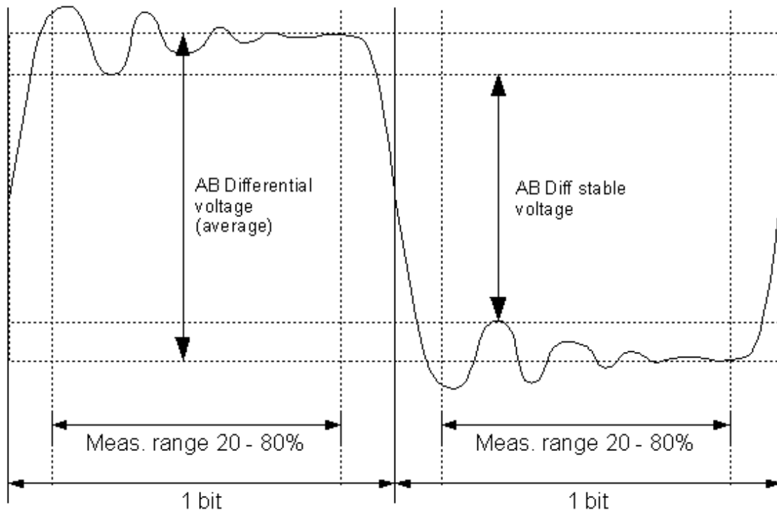
Abb. 26 - Messprinzip der Balkendiagramm-Modi
