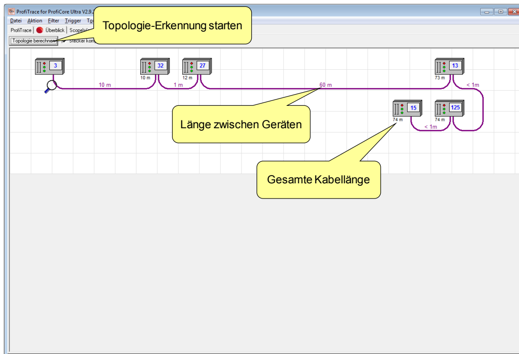
Abb. 6 - Topologie-Erkennung
