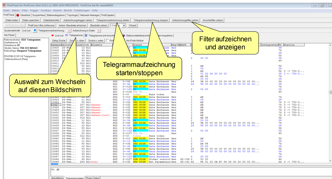
Fig. 18 - ProfiTrace Telegrammaufzeichnung
