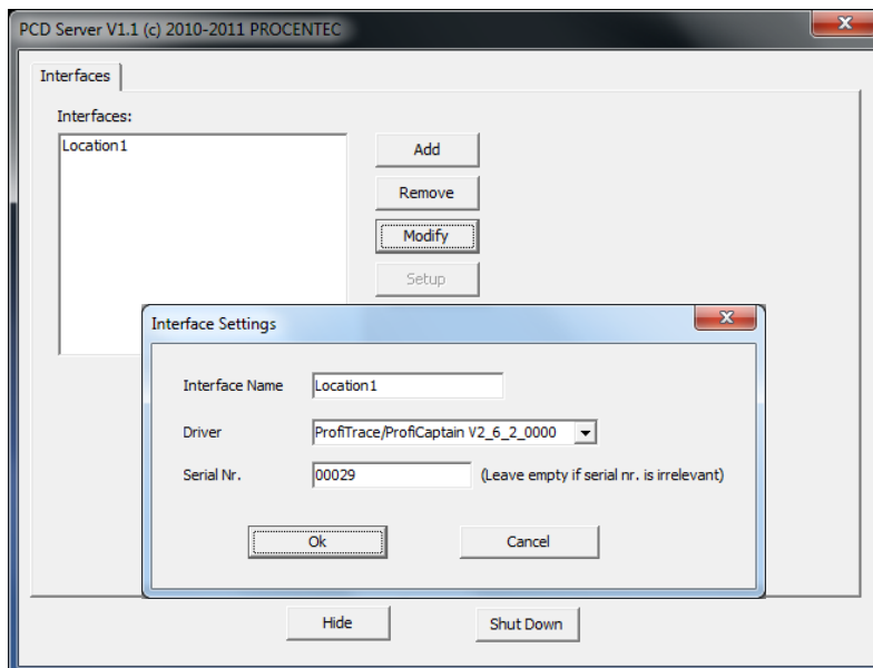
Abb. 17 - PCD-Server einrichten
