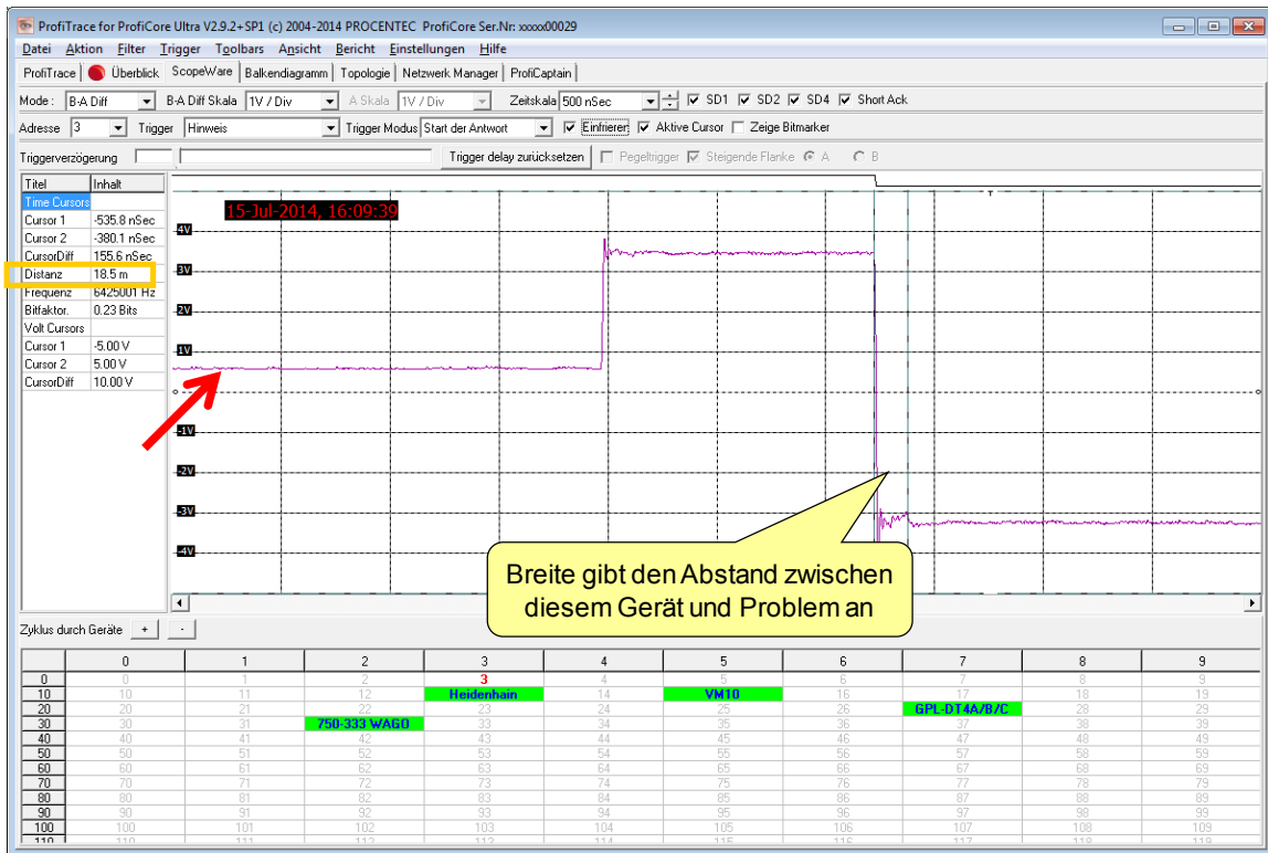
Abb. 42 - Passive Terminierung
