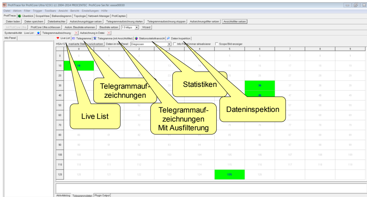
Abb. 4 - ProfiTrace-Funktionen
