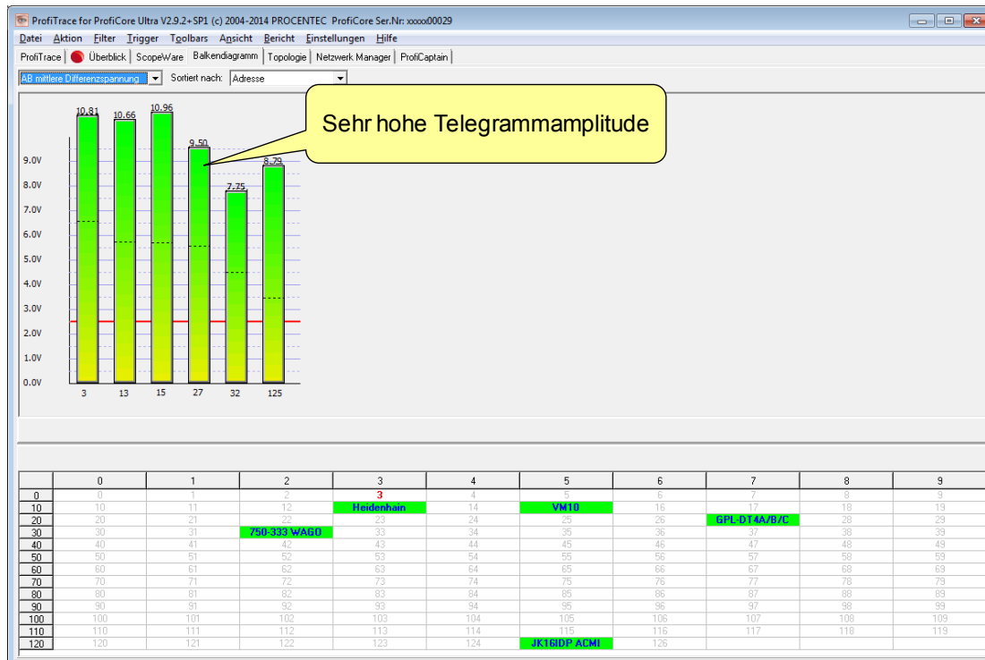
Abb. 23 - Balkendiagramm, wenn fehlende Terminierung oder ein Kabelbruch erkannt
