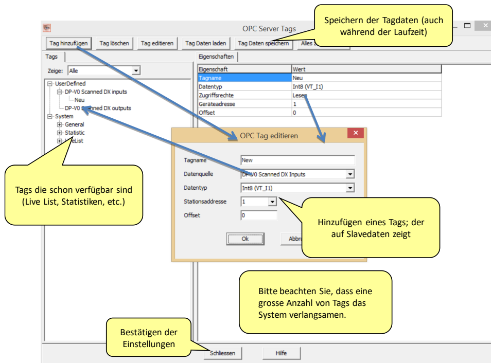
Abb. 49 - OPC-Tags hinzufügen
